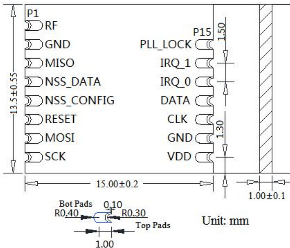
图 3-2 LSD4RF-2H310N10 模块外形尺寸图
